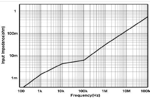
图 3.c HCP8030D 输入阻抗 VS 频率曲线
