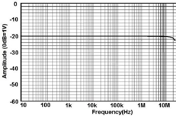
图 7.b HCP8150A 幅频曲线
