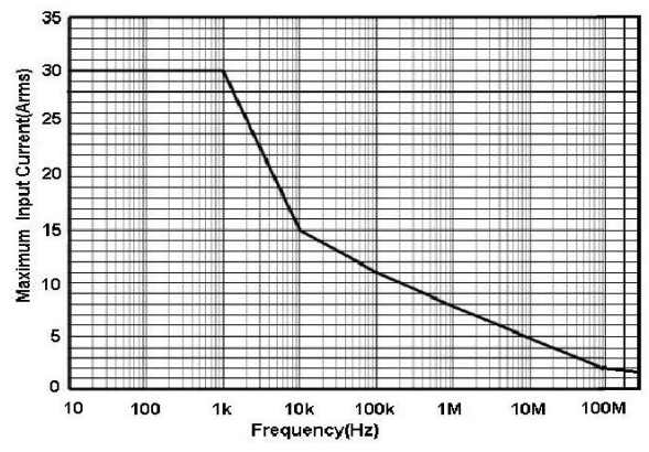
图 2.d HCP8030H 最大测量电流 VS 频率曲线 (超过该曲线所示最大电流连续使用会导致探头烧毁)
