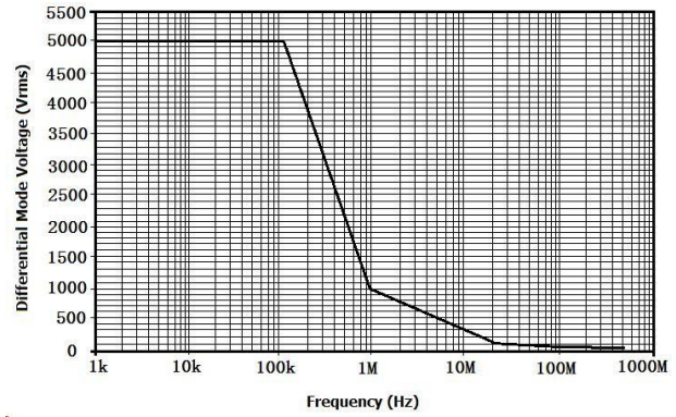
图 4 DP6700A 最大差模电压 VS 频率
