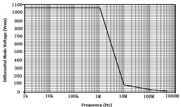
图 2 DP6150A 最大差模电压 VS 频率
