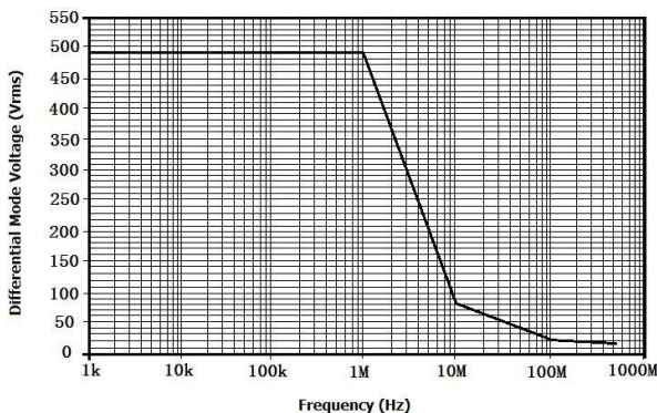
图 1 DP6070A 最大差模电压 VS 频率
