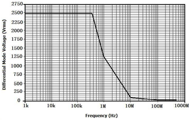
图 3 DP6350A 最大差模电压 VS 频率
