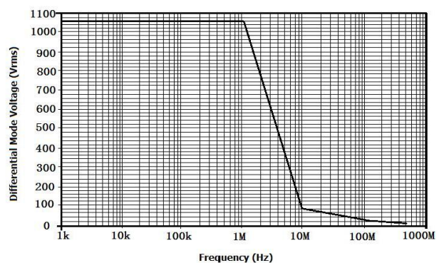
图 2 DP6150B 最大差模电压 VS 频率
