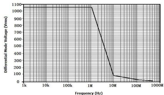
图 2 DP6150D 最大差模电压 VS 频率
