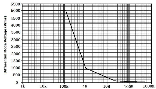
图 4 DP6700D 最大差模电压 VS 频率
