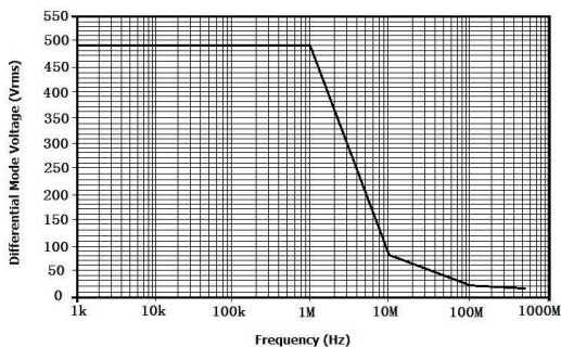
图 1 DP6070D 最大差模电压 VS 频率
